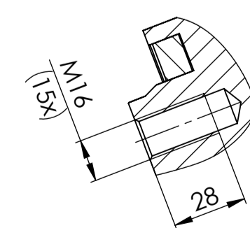
SCHNITT A-A
