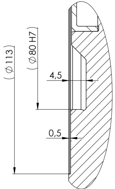
DETAIL A MAßSTAB 2 : 1
